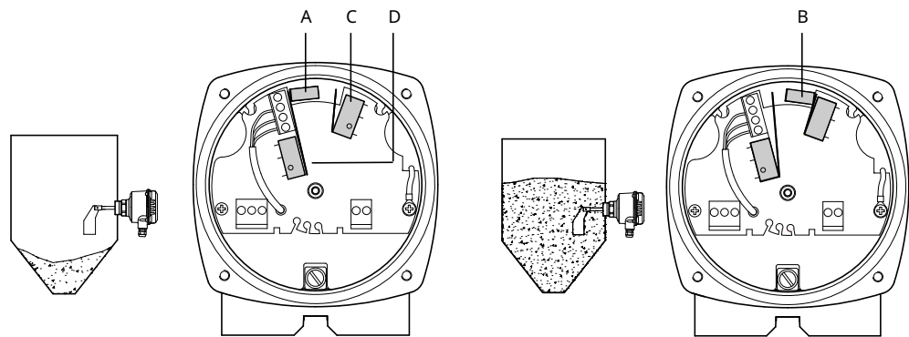
Figure 1: Switching Lug Function
